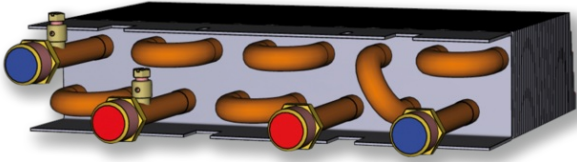
Échangeur de chaleur avec système à 4 tubes
