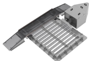
DECKENKLAPPE MIT EINBAURAHMEN, WÄRMEEINHAUSUNG UND ÜBERGANG
