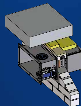
Einbausituation gleitender Deckenanschluss
