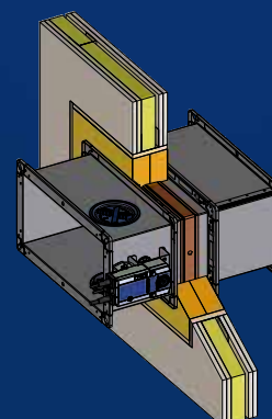
Einbausituation Weichschott
