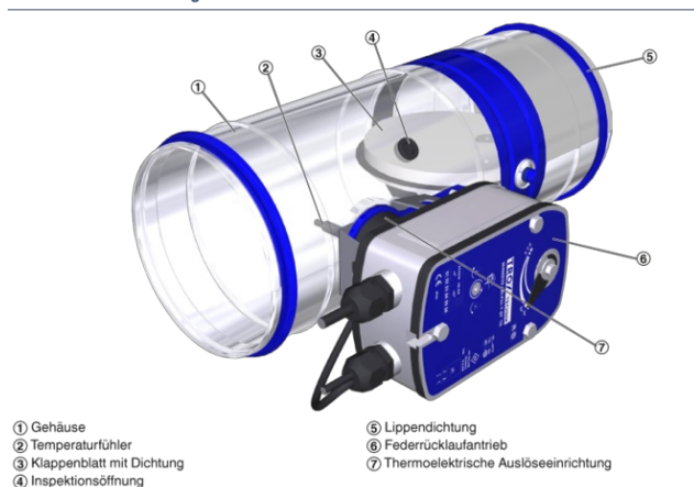
Schematische Darstellung FKRS-EU mit Federrücklaufantrieb
