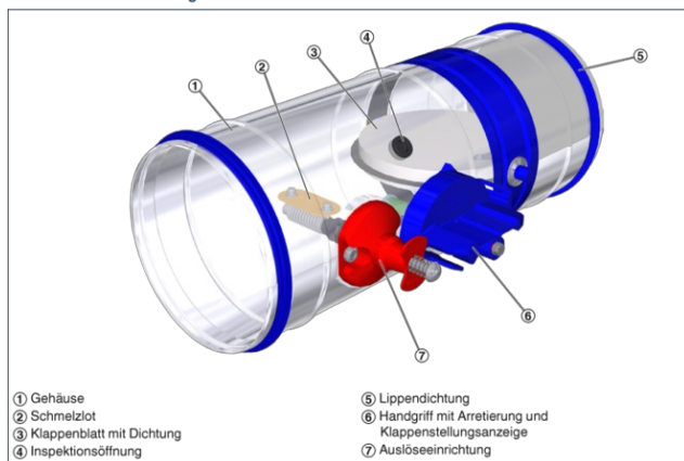
Schematische Darstellung FKRS-EU mit Schmelzlot
